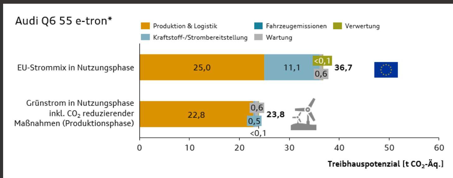
Abbildung 2: Treibhauspotenzial des Audi Q6 55 e-tron quattro* über den gesamten Lebenszyklus
